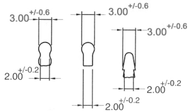
Détail A
